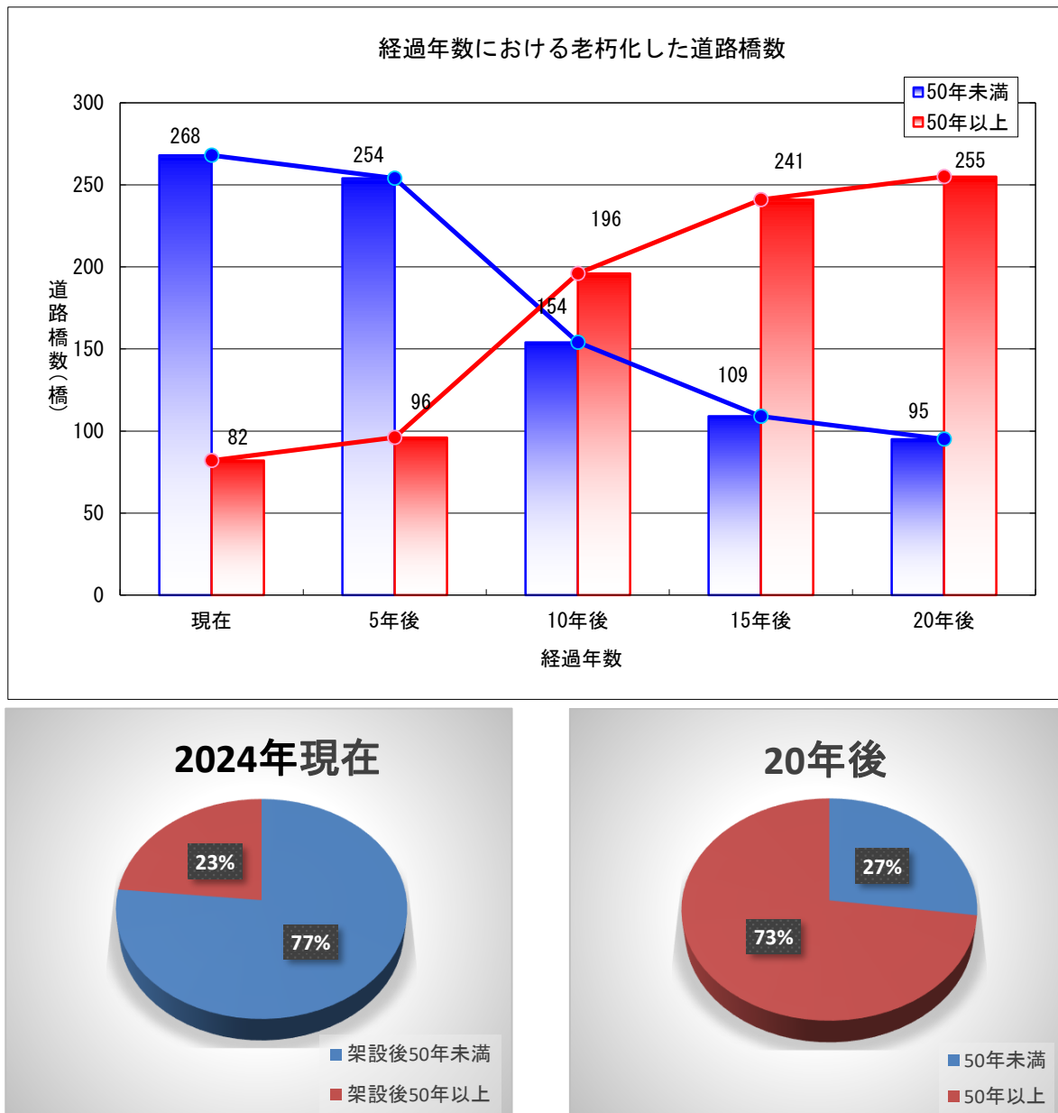
図3-1 建設後50年以上経過した道路橋数の変化
