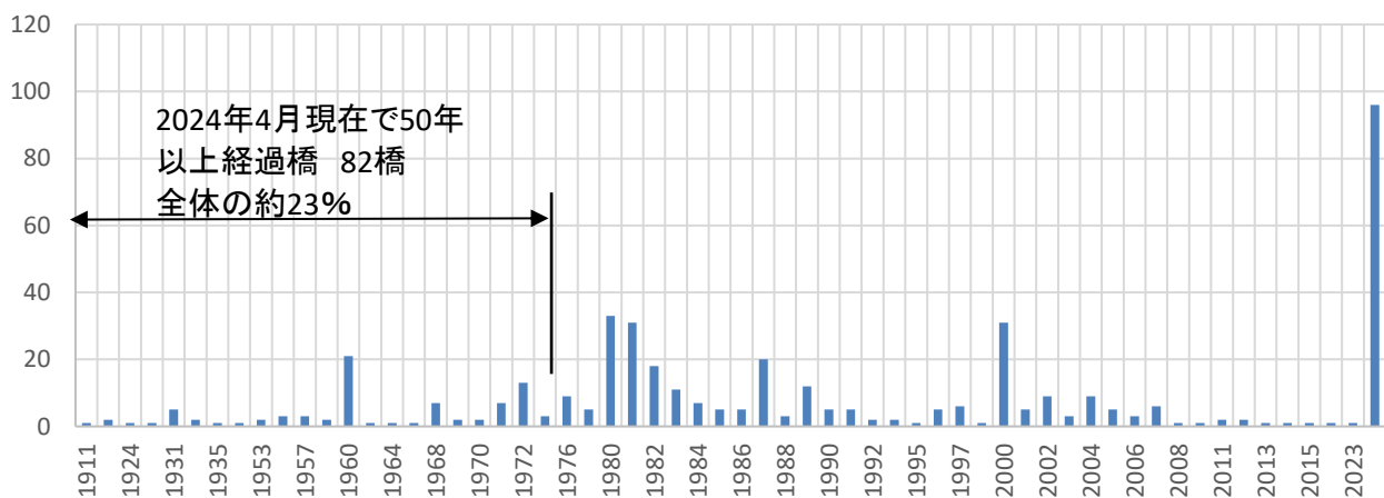
架設年次別橋数
