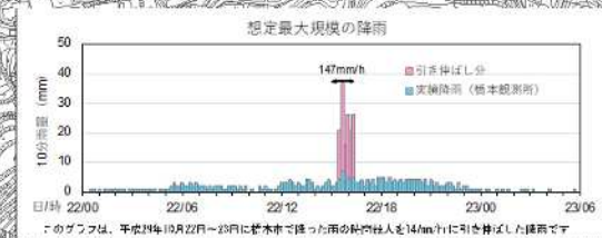
橋本市内水浸水想定区域図（浸水継続時間）図郭⑩【想定最大規模降雨】
