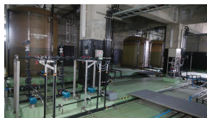
薬品注入設備（ポリ塩化アルミニウム、苛性ソーダ）
