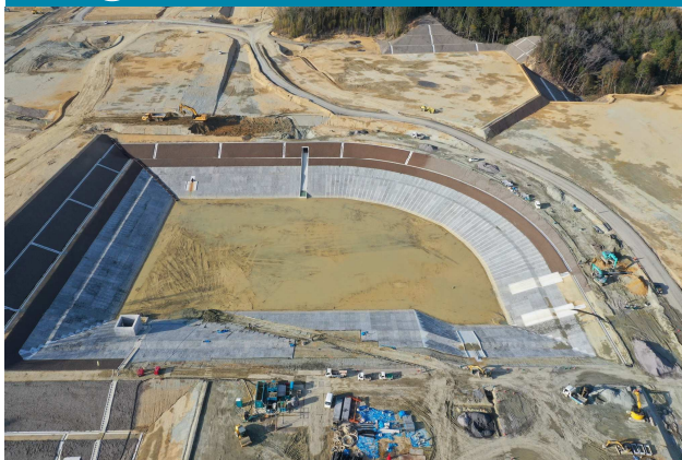
⑥ 1号調整池の施工状況
