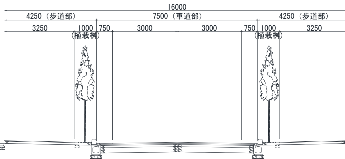
山内垂井線 標準断面図
