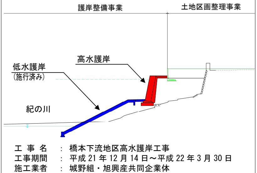
標準断面図
