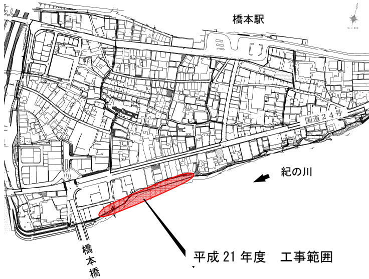
工事位置図
